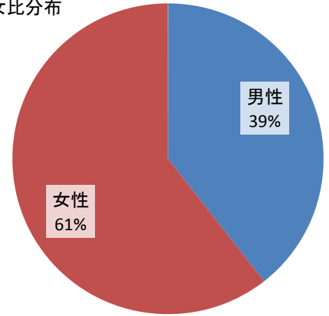
図3 男女比分布
