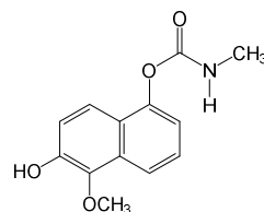
代謝物AA
