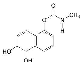
代謝物H
