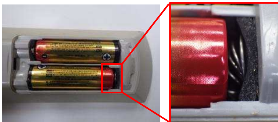
(写真2) ばね端子を介したアルカリ乾電池のショート（イメージ）
